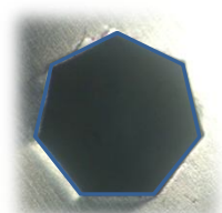
Heptagon Siebener Heptágono
