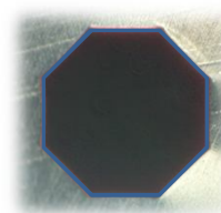
Octagon Achteck Octágono
